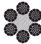
6x26WS Dycam
